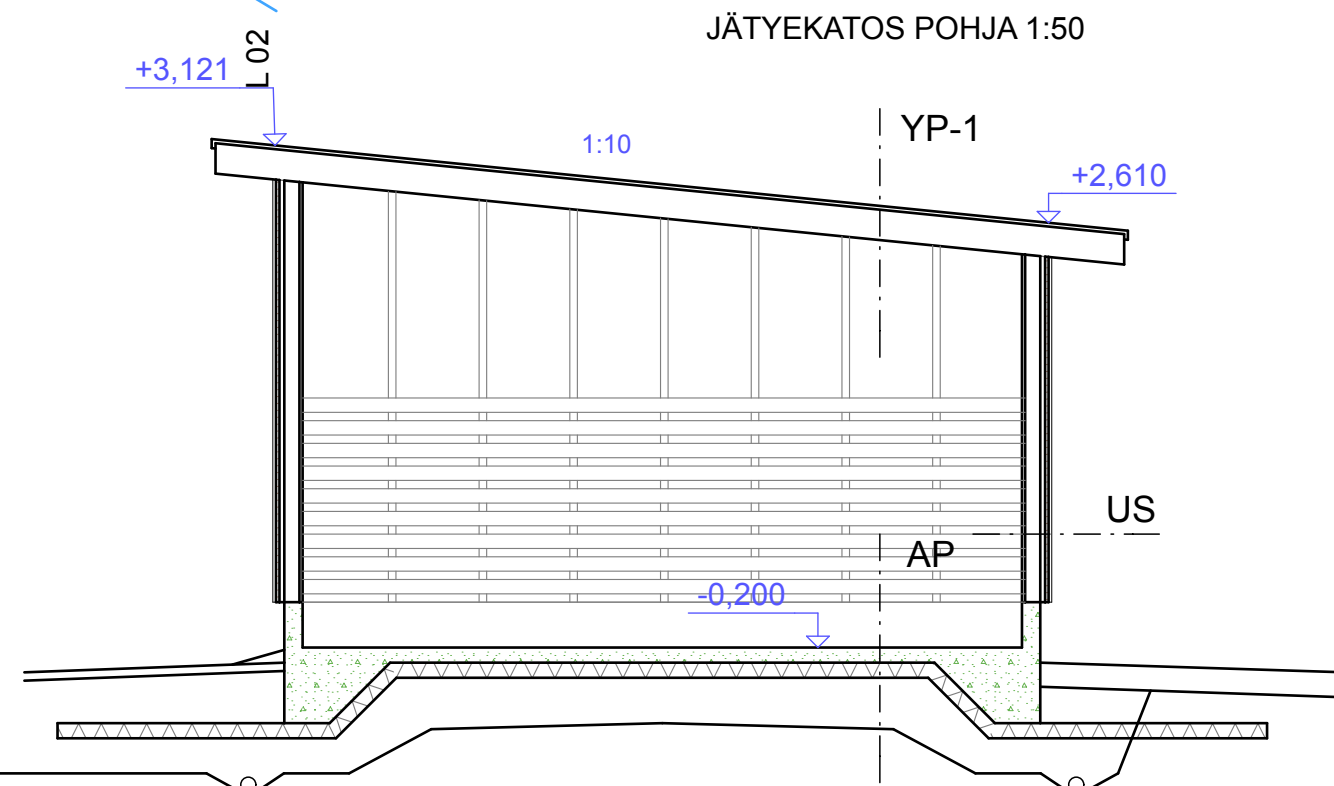
JÄTEKATOS LEIKKAUS L02-L02 1:50
