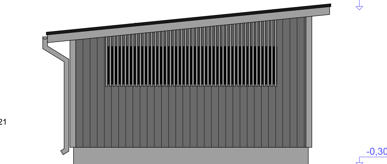
JÄTEKATOS JULKISIVU LOUNAASEEN 1:50
